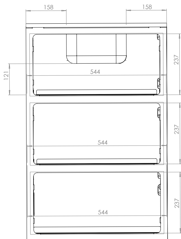
Wymiary modułu w wersji z półkami (drzwiczkami) Dimensions of module with shelves (door)
