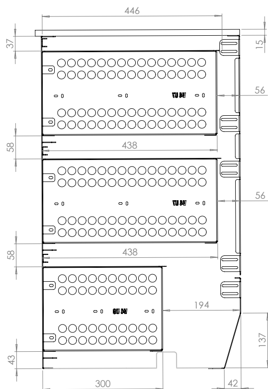
Wymiary przy maksymalnym rozsunięciu tylnej blachy
