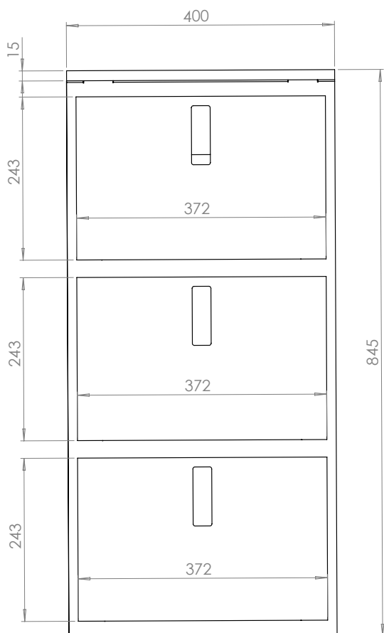
Wymiary wariantu z szufladami Version with drawers
