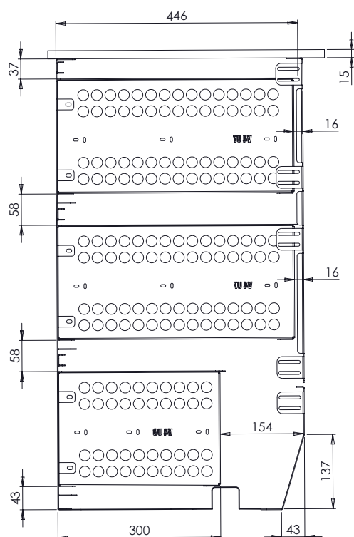
Wymiary przy maksymalnym zsunięciu tylnej blachy
