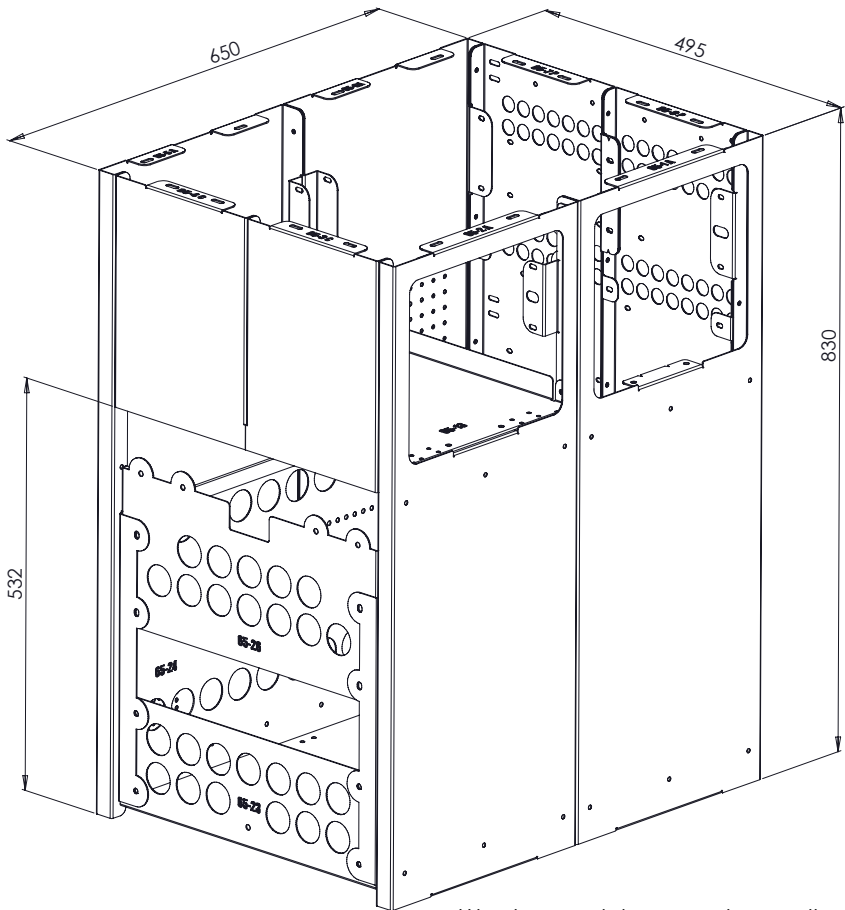
Wymiary modułu, rzut w izometrii Module dimensions, projection in isometry
