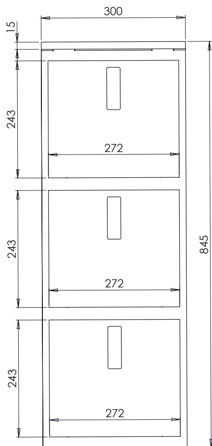
Wymiary wariantu z szufladami Version with drawers
