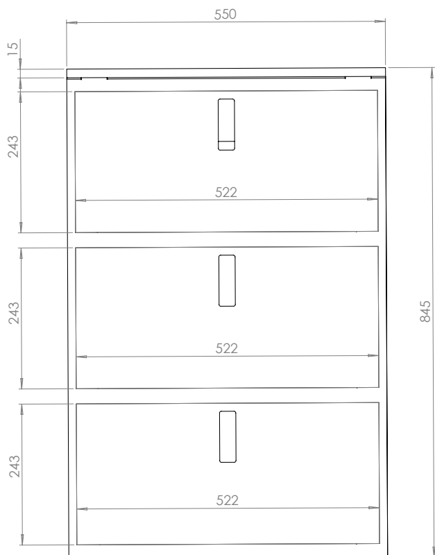
Wymiary wariantu z szufladami Version with drawers
